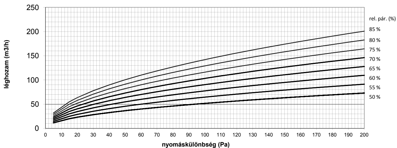
GBP 444 típusú légvezetők jelleggörbéje a nyomáskülönség és a páratartalom függvényében
