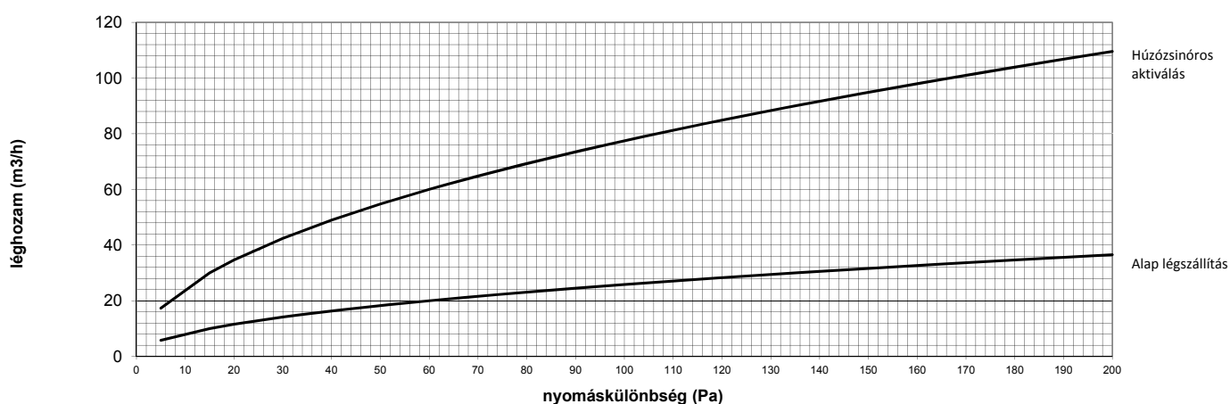
GBP 443 típusú légvezetők jelleggörbéje a nyomáskülönség függvényében
