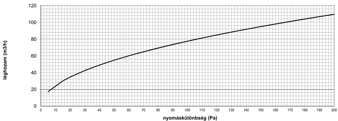
GBP 480 típusú légelvezetők jelleggörbéje a nyomáskülönbég függvényében
