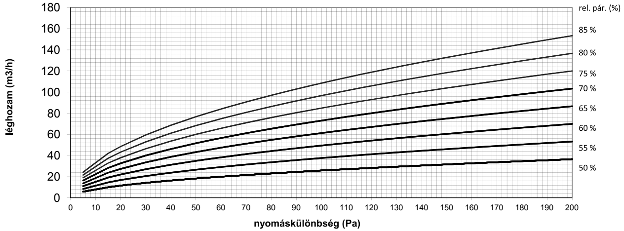
GBP 479 típusú légelvezetők jelleggörbéje a nyomáskülönbég függvényében
