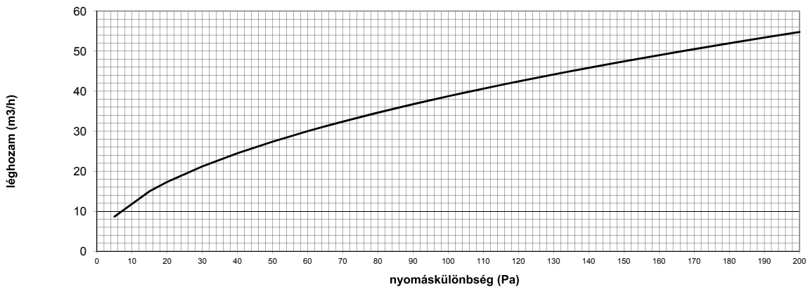
GBP 479 típusú légelvezetők jelleggörbéje a nyomáskülönbég függvényében
