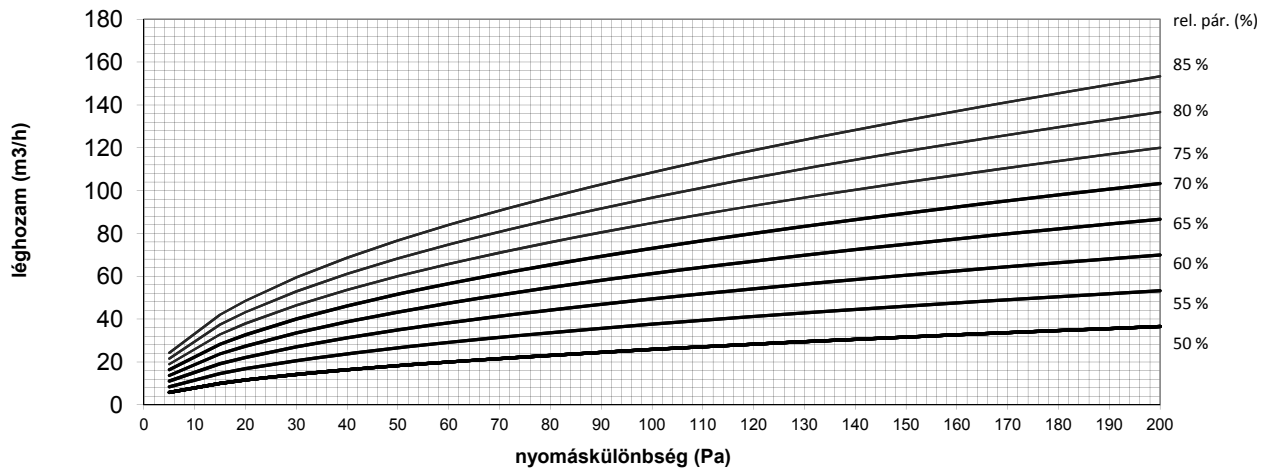
GBP 479 típusú légelvezetők jelleggörbéje a nyomáskülönbség függvényében
