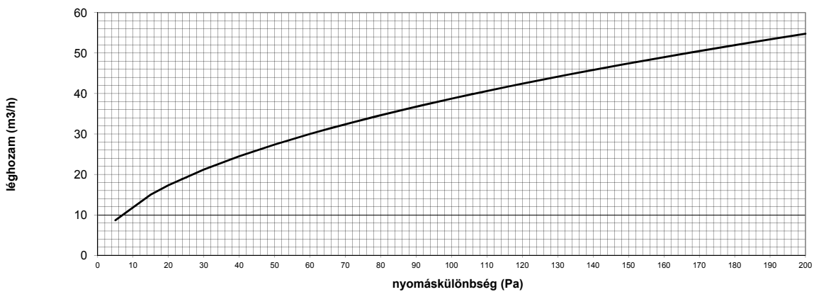
GBP 479 típusú légelvezetők jelleggörbéje a nyomáskülönbség függvényében
