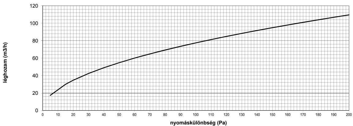
GBP 480 típusú légelvezetők jelleggörbéje a nyomáskülönbség függvényében
