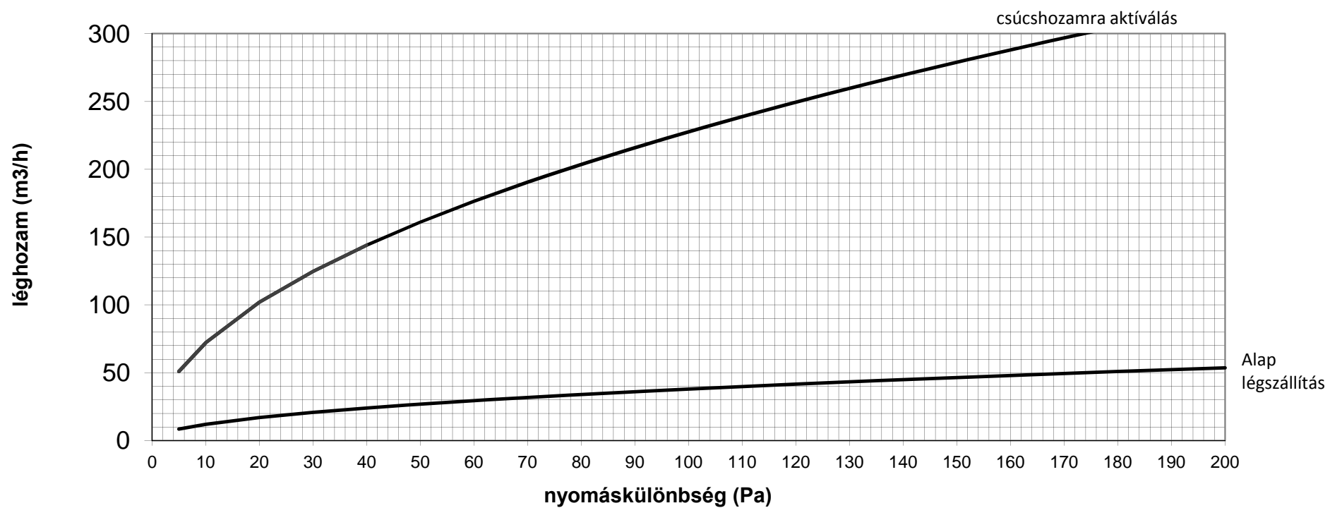
G2H 1070 kapcsolóval rendelkező légelvezető jelleggörbéje a nyomáskülönbség függvényében
