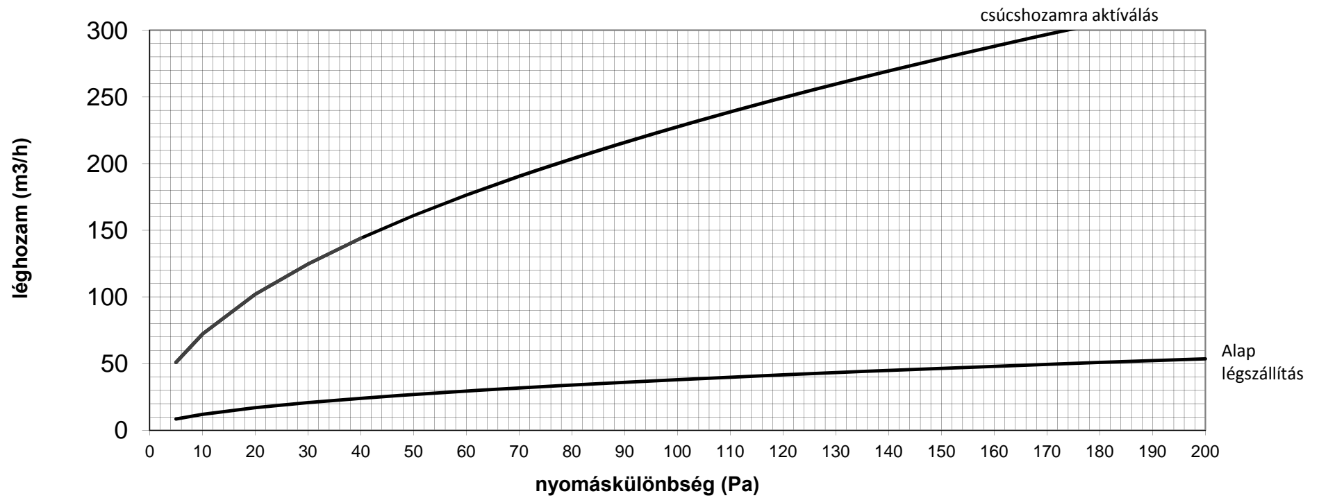
G2H 1069 mozgásérzékelővel rendelkező légvezető jelleggörbéje a nyomáskülönbség függvényében
