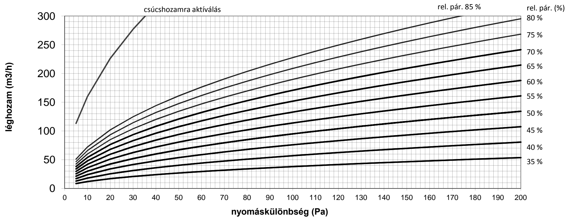
G2H 1068 típusú higroszabályozású és távirányítóval kapcsolható légelvezető jelleggörbéje a nyomáskülönbség és a páratartalom függvényében
