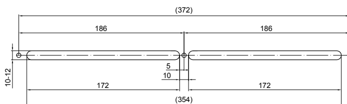
1. ábra A szükséges szellőzőrés méretei
